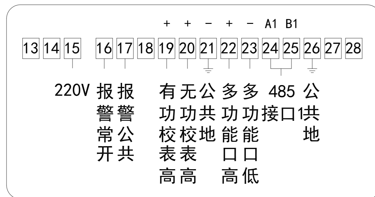
外拉有源220V交流输出、一路485
