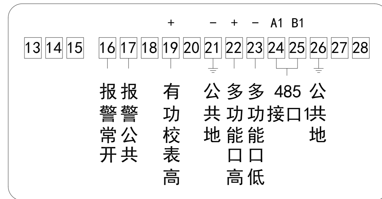
带报警、一路485
