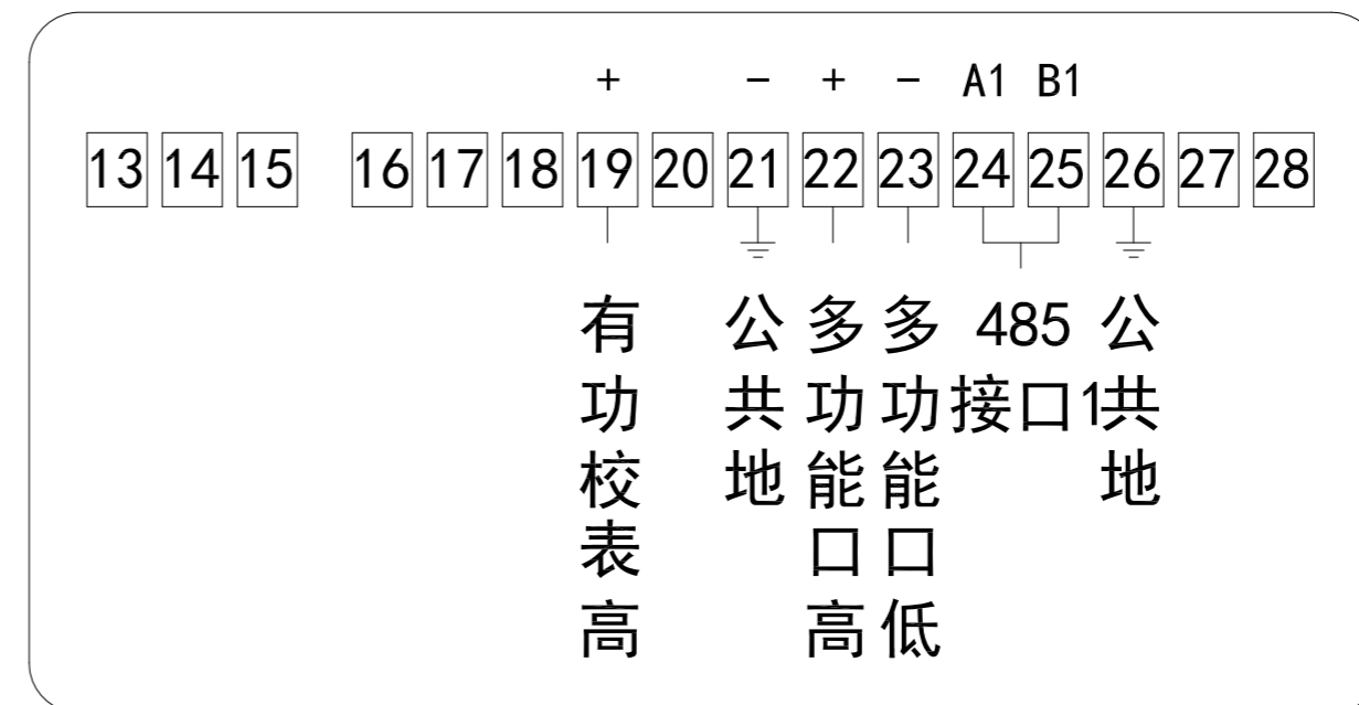
一路485
