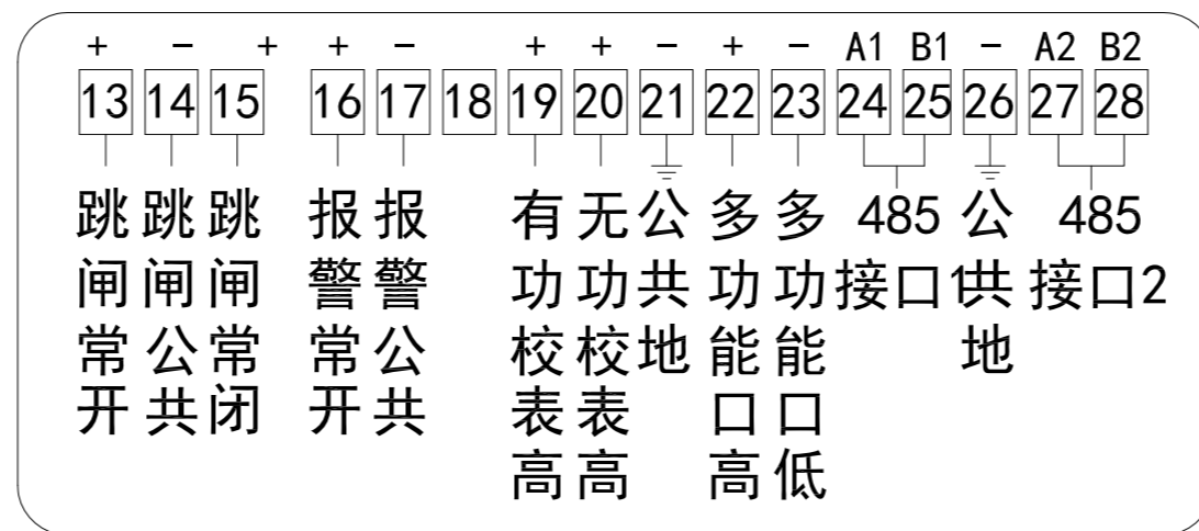
二路485
