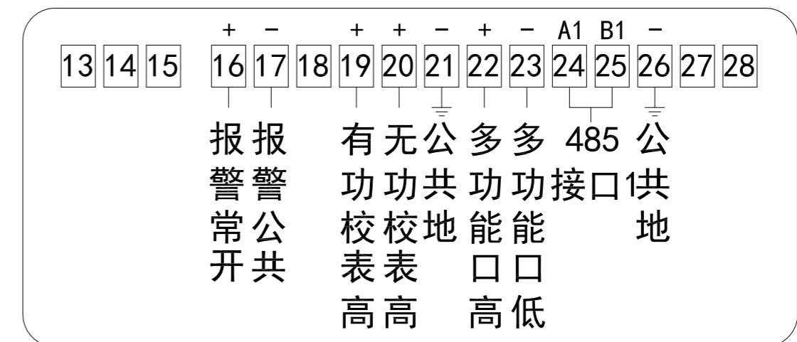
内置拉合闸
