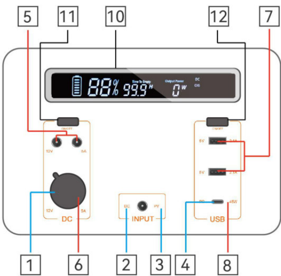
主视图
