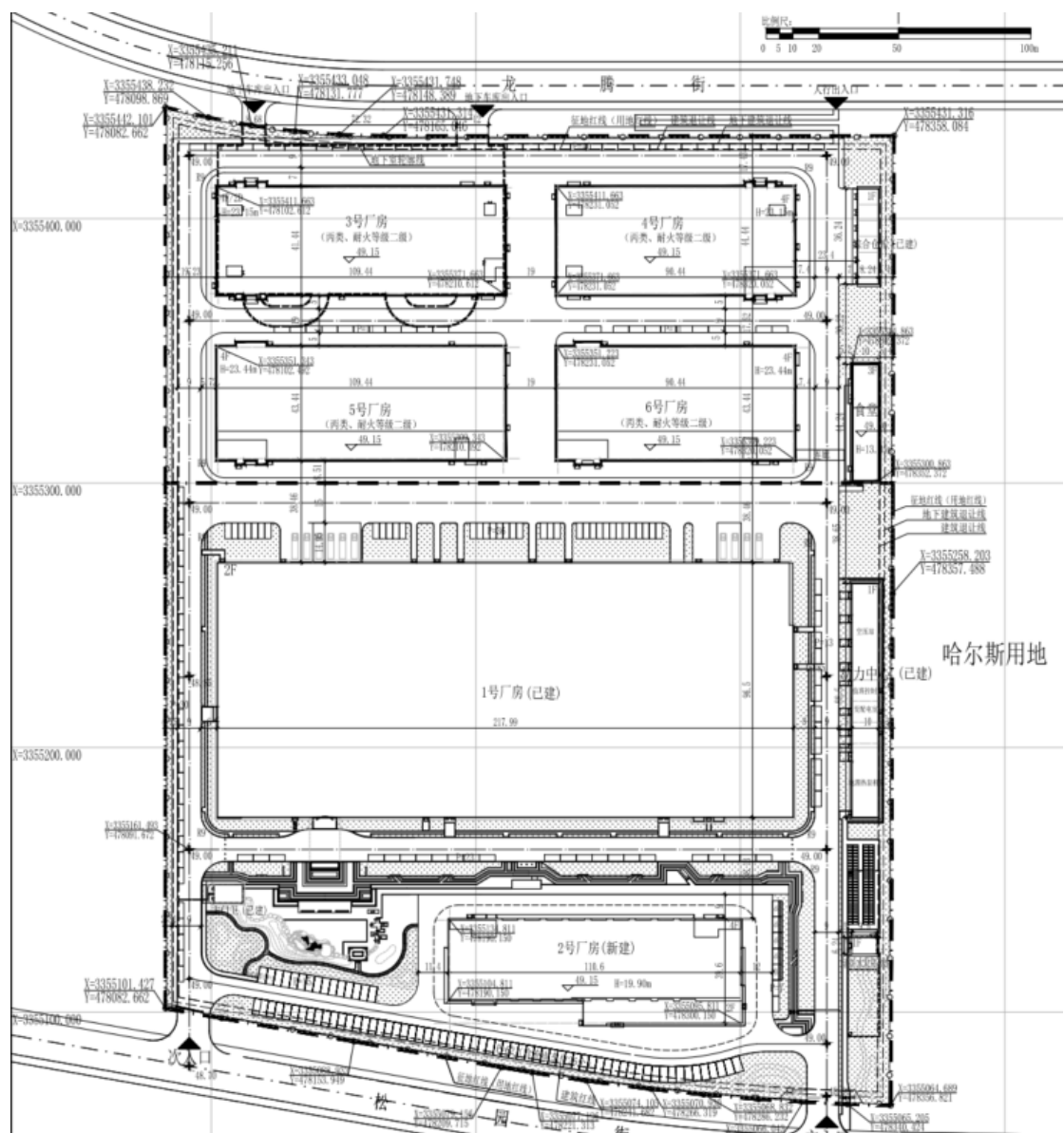
图 3.4 平面布局图
